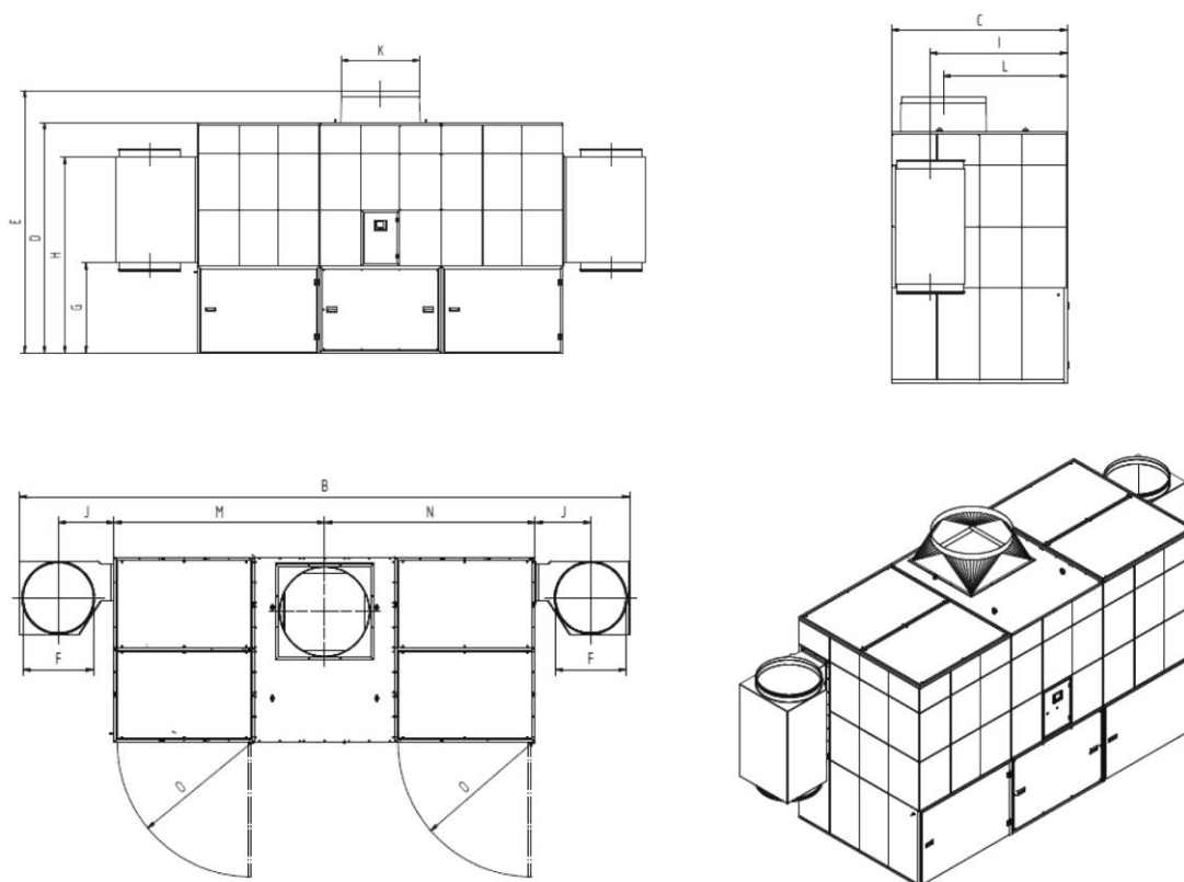
Obr. 77: Rozměrový výkres 34160
