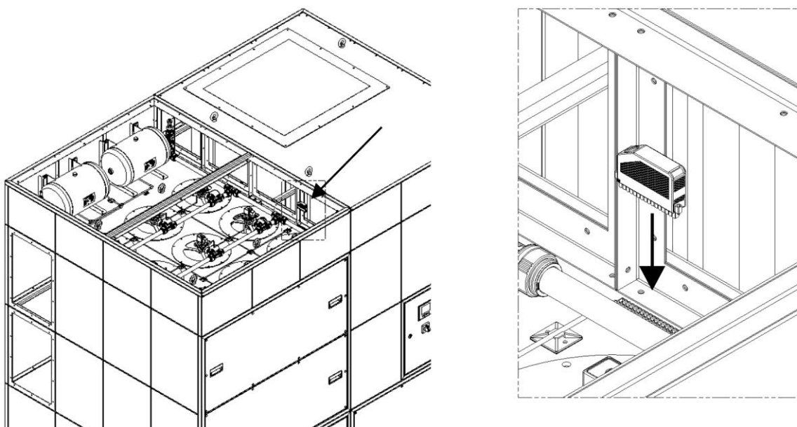
Obr. 22: Montáž zelené zástrčky
