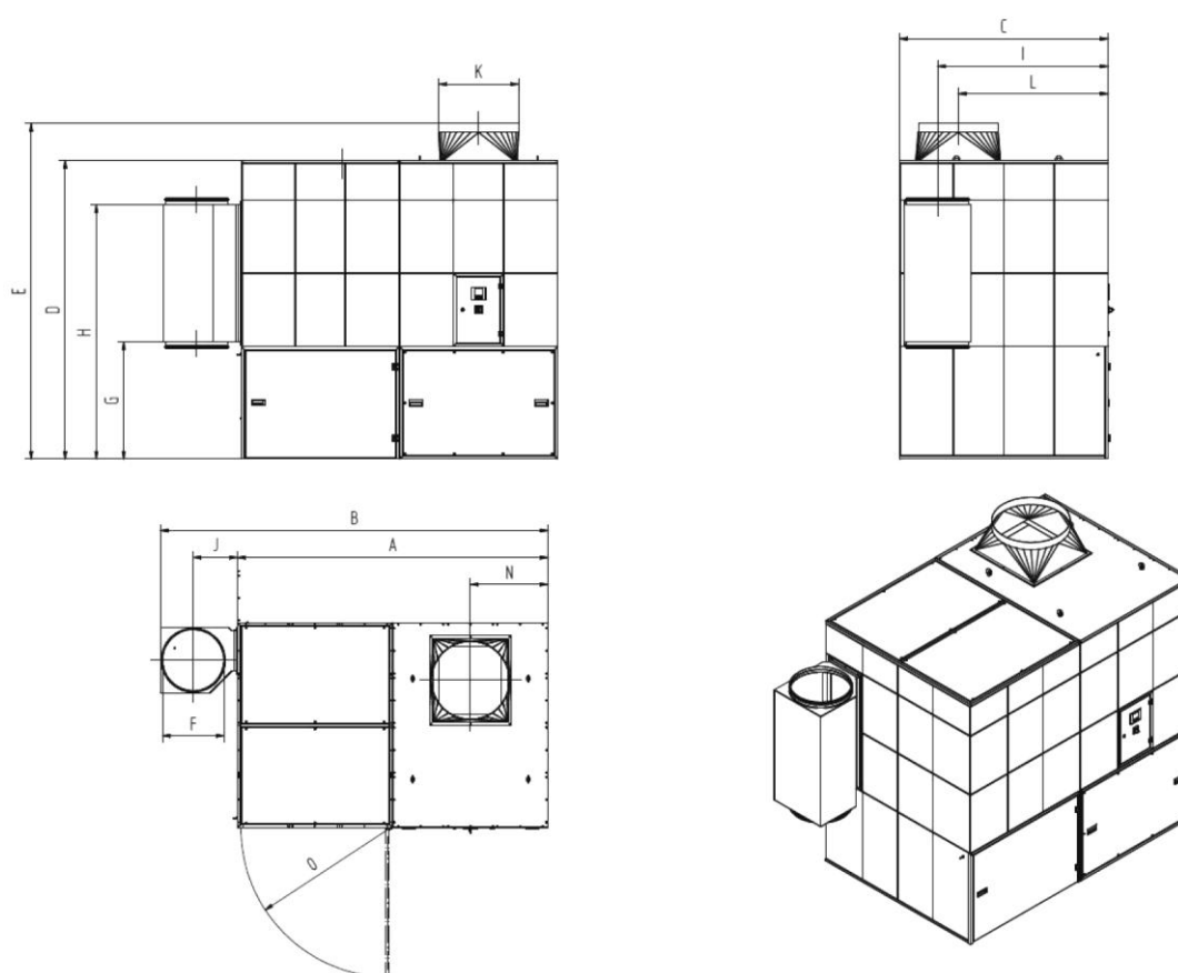
Obr. 76: Rozměrový výkres 34130
