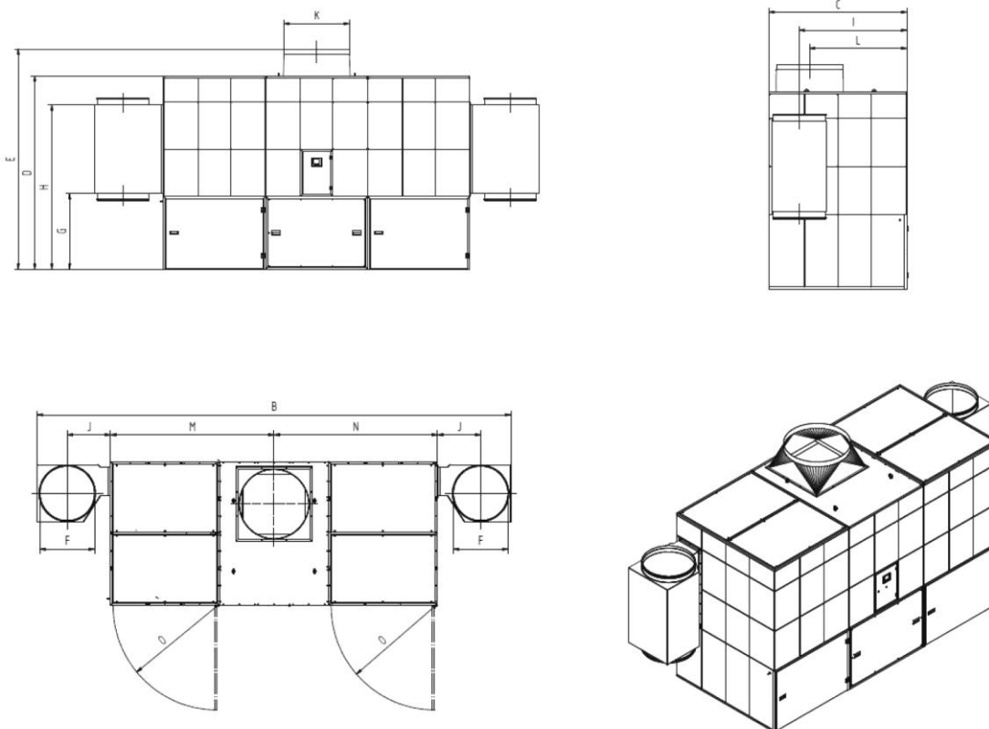
Obr. 78: Rozměrový výkres 34180
